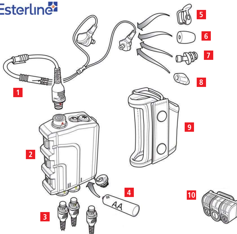
■ Hlavní části systému: 1 – náhlavní souprava ELITE; 2 – přepínací jednotka; 3 – radiokabely; 4 – baterie; 5 – ucpávka Concha hook; 6 – pěnová ucpávka; 7 – gumová ušní ucpávka; 8 – silikonová ušní ucpávka; 9 – pouzdro; 10 – bezdrátové tlačítko klíčování
